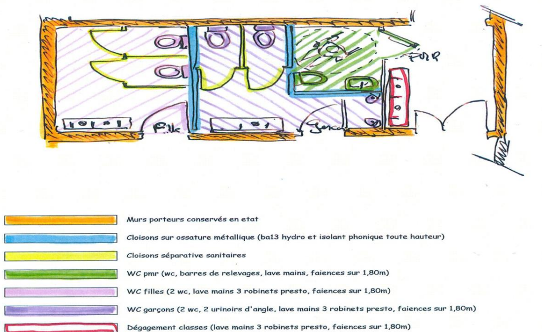
Plan de localisation et schéma de principe des travaux
